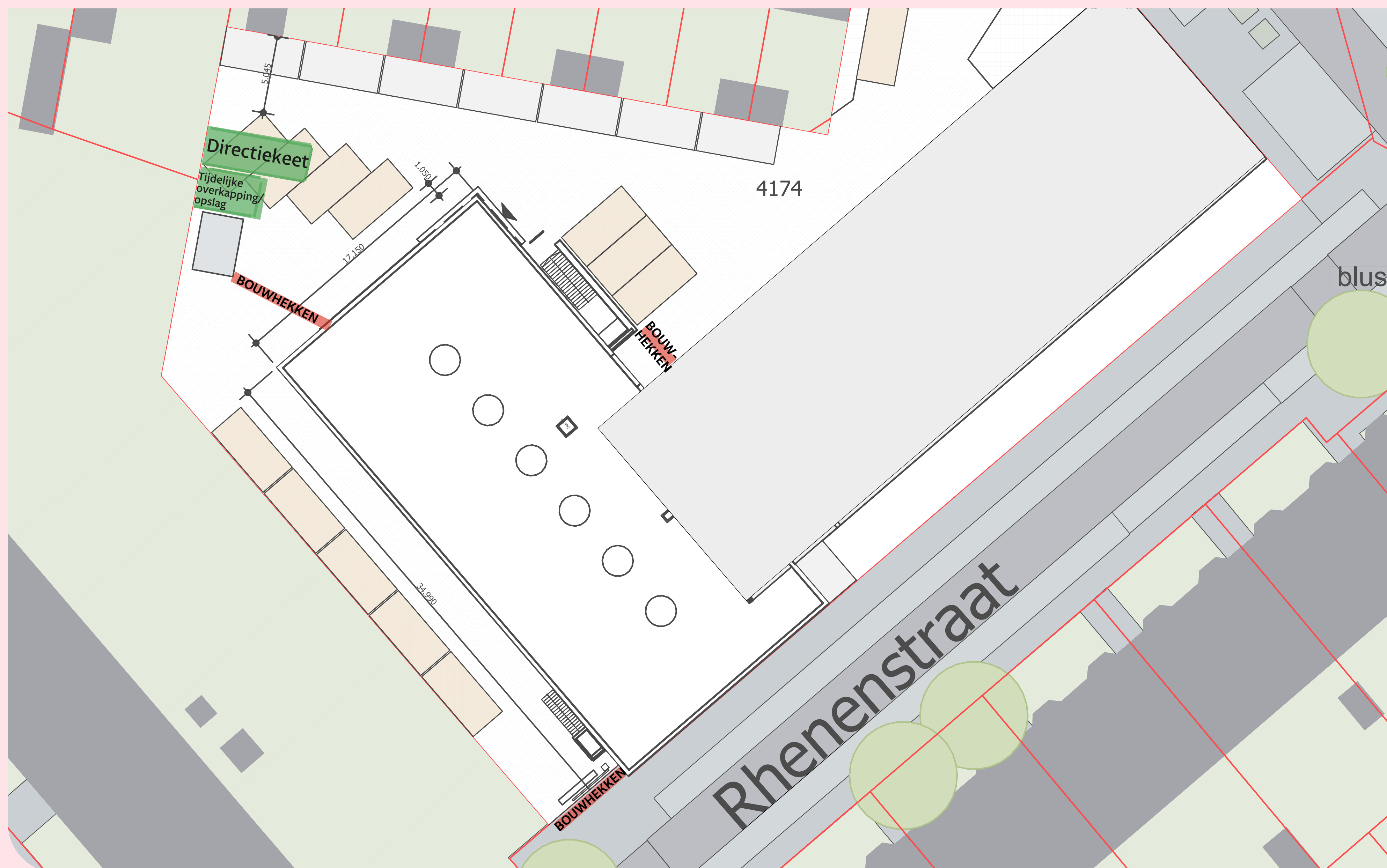
Inrichting bouwplaats
